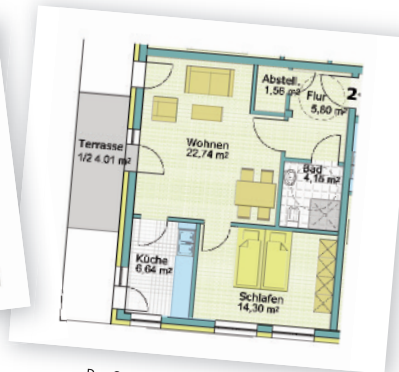
Der Grundriss zeigt eine Wohnung im Betreuten Wohnen.
