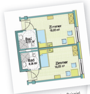
Der Grundriss zeigt das Beispiel eines 1-Bett-Pflegezimmers mit einer Größe von 22 m 2 .
